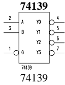
74139
