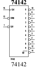
74142
