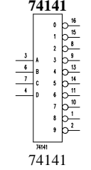
74141
